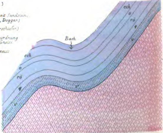
Fig. 7. Übersprünge der Schieferung vom Glimmerschiefer auf den Verrucano ob der Spitzgrassenplattge am Fuss des Schlossbergs
